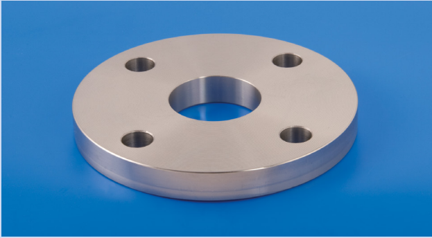
FLANGE EN 1092-1 TYPE 01
